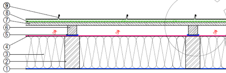
Рис.4 Конструкция крыши с металлической кровлей, ОДМ и диффузионной мембраной, уложенной на утеплитель. Фальцевая кровля смонтирована на ОДМ поверх сплошного настила.
